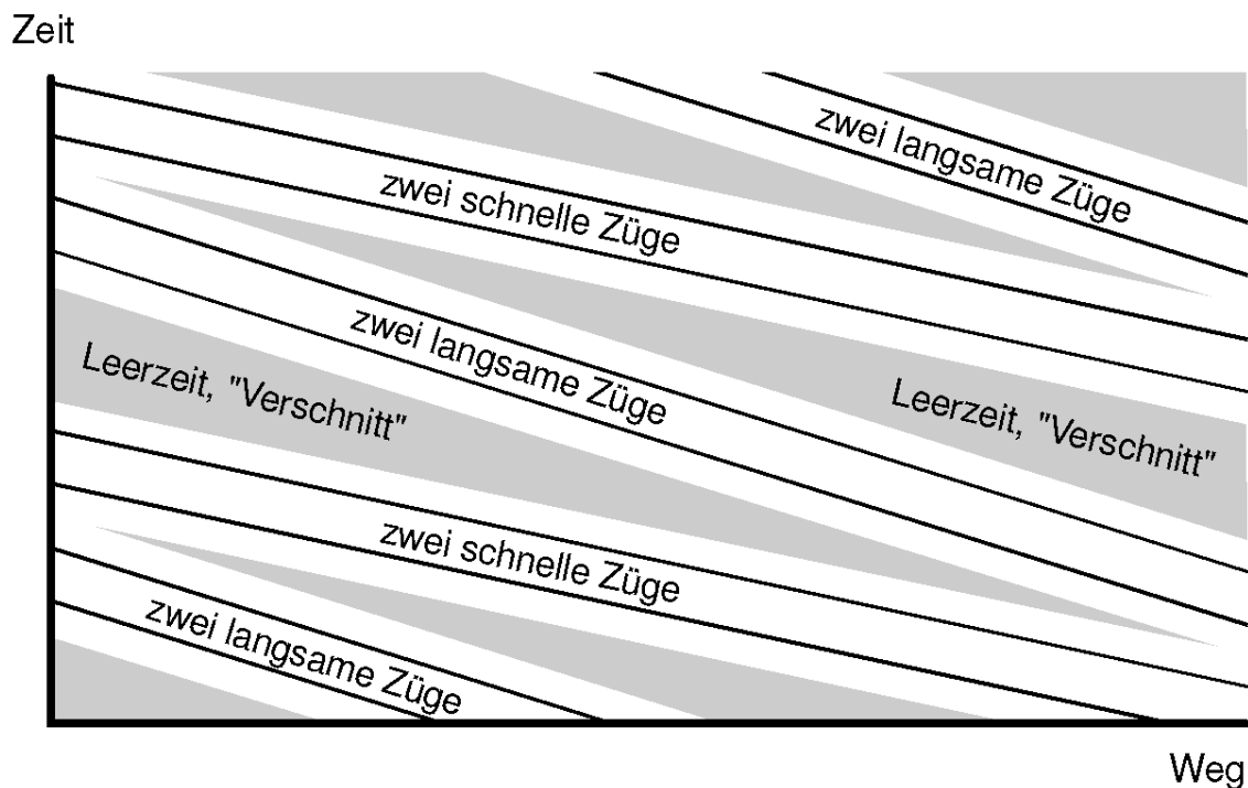
Abb. 5: Beispielhafter Bildfahrplan mit unterschiedlichen Zuggeschwindigkeiten
