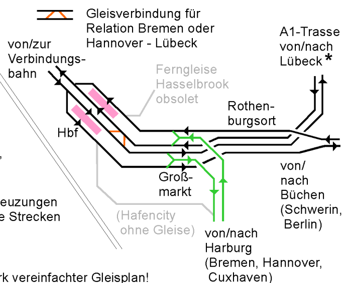
Abb. 4: (links) Heutiger Gleisplan mit betrieblichen Einschränkungen und (rechts) künftiger Gleisplan ohne Einschränkungen mit A1-Neubaustrecke statt S4-Ausbaustrecke
