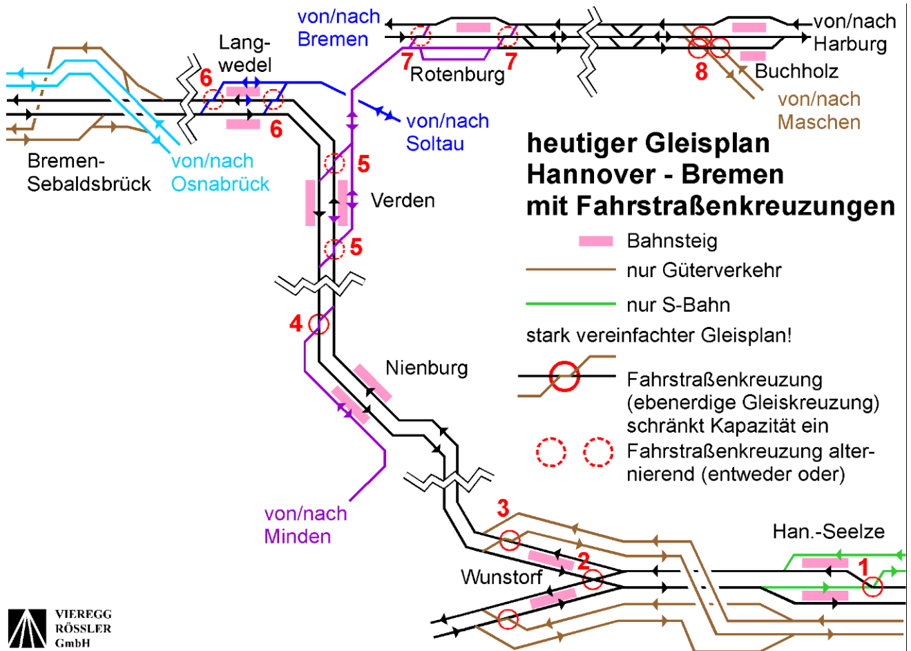
Abb. 6: Stark vereinfachter Gleisplan Hannover - Bremen im heutigen Zustand mit Darstellung der Fahrstraßenkreuzungen
